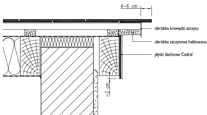
Wykonanie szczytu z płytką maskującą oraz blachą
