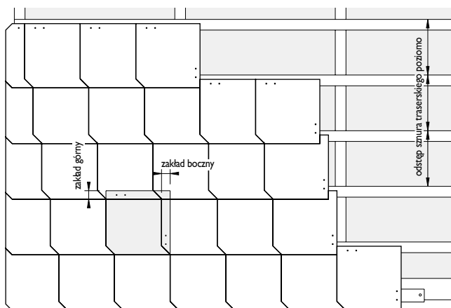
Przykład: Format 30 x 30 cm, ze ściętymi rogami, z docinaniem kryciem szczytu
