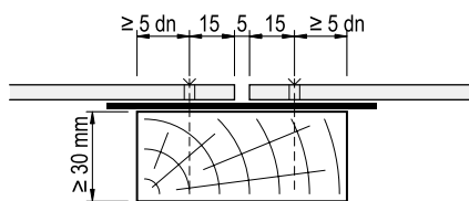
Wykonanie szczelin
