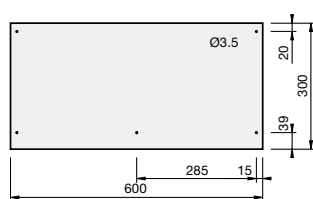
60 x 30 cm, 5 otworów
